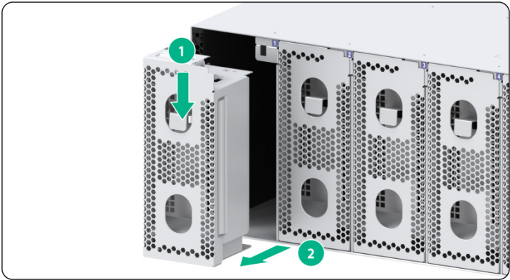
图2-25 接口模块扩展卡假面板拆卸示意图
