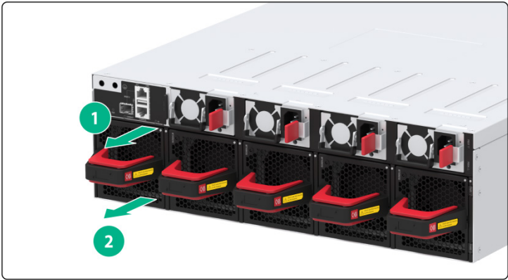
图2-17 FAN-80B-1-B-Z-Z 风扇模块拆卸示意图
