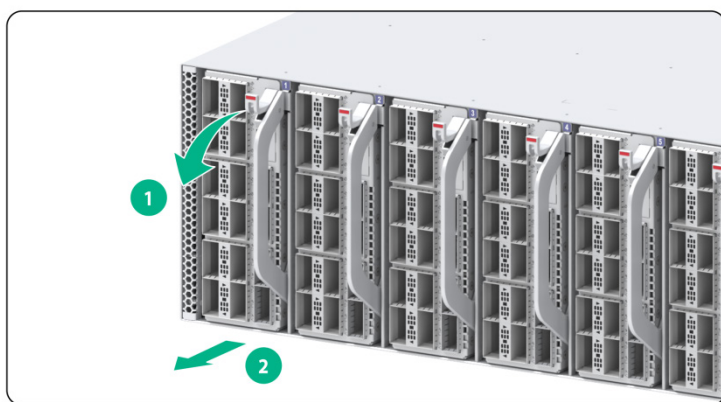
图2-28 接口模块扩展卡拆卸示意图
