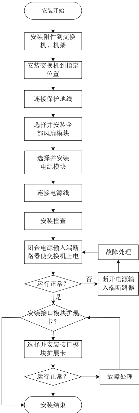
图2-1 交换机安装流程
