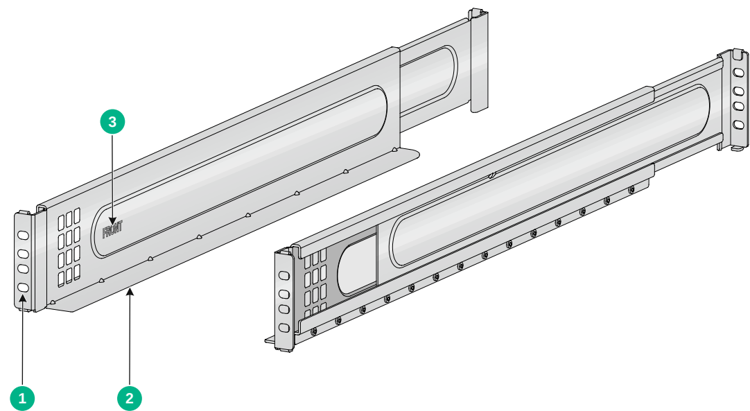
图2-6 S9600XP-8C-G 滑道示意图
