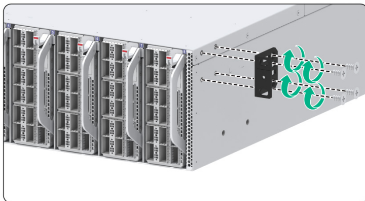
图2-8 安装挂耳到 S9600XP-8C-G 机箱的示意图
