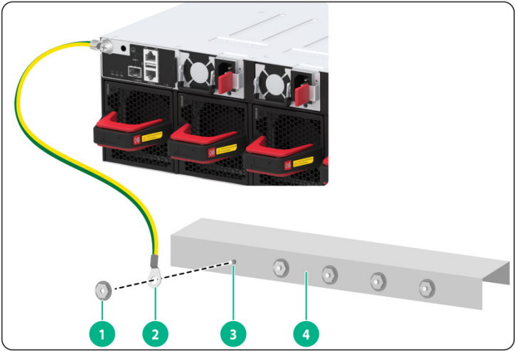
图2-14 连接接地线缆到接地排
