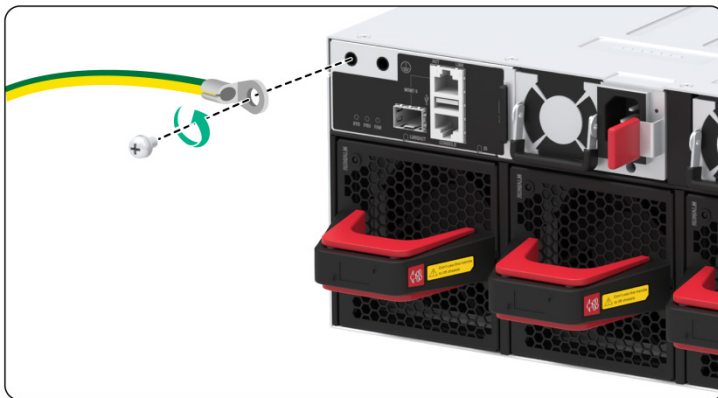
图2-13 安装接地线到 S9600XP-8C-G 接地点示意图
