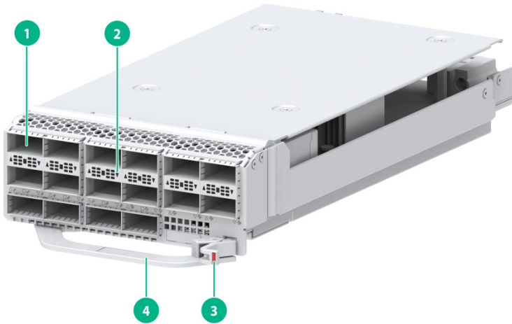
图2-26 LSWM1CGQ16M1-Z 接口模块扩展卡外观图
