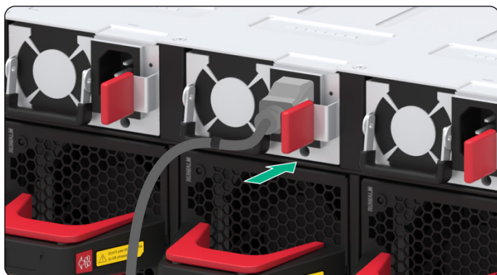
图2-24 PSR1300-12A-C-A-Z-Z 交流电源线连接示意图
