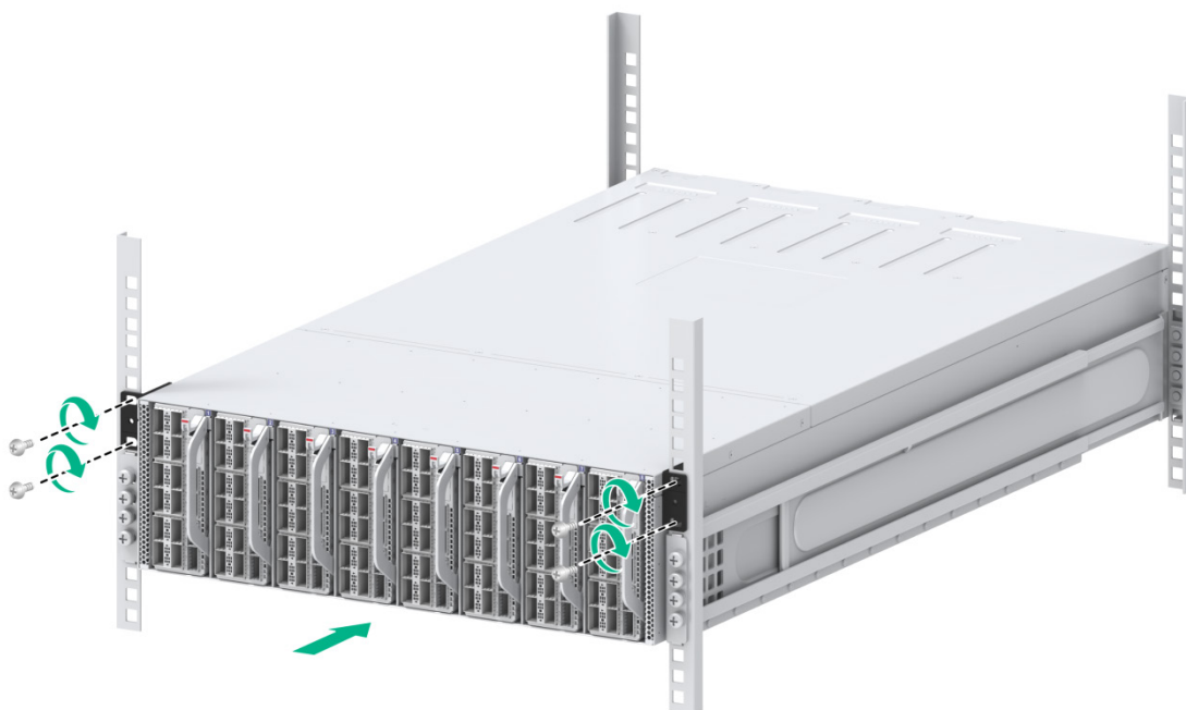
图2-10 安装 S9600XP-8C-G 交换机到机柜示意图
