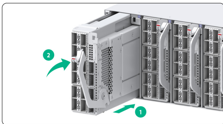
图2-27 接口模块扩展卡安装示意图
