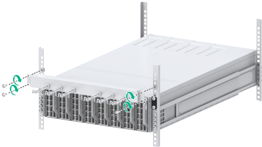
图2-11 安装走线架到机柜示意图
