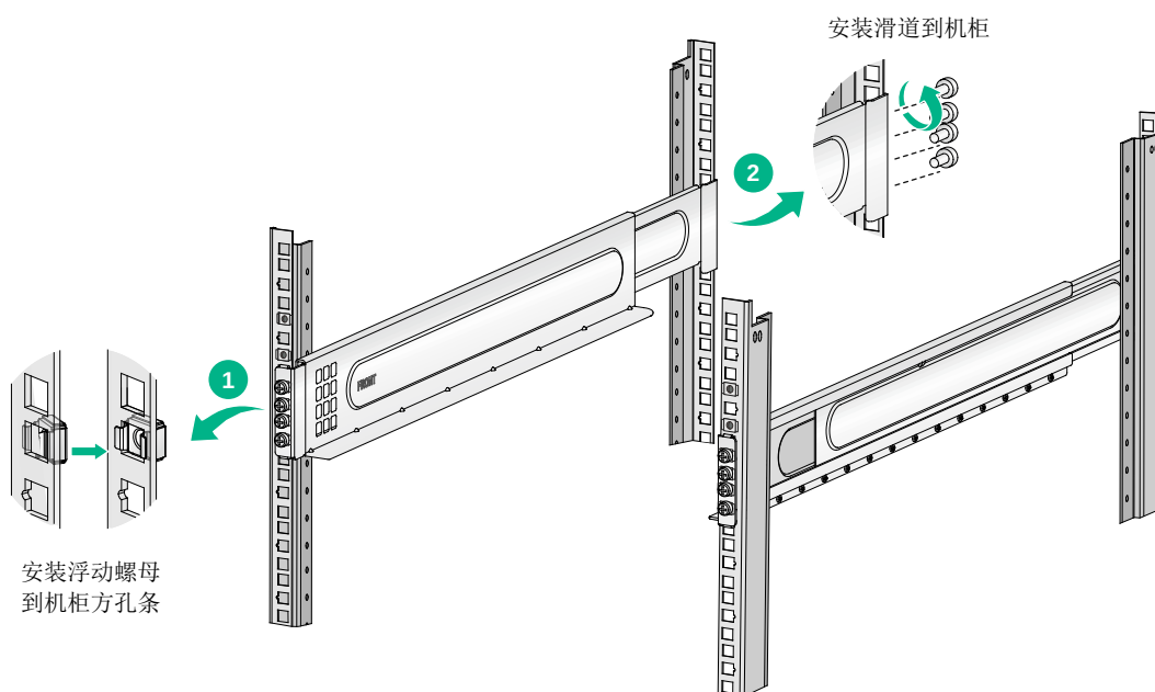
图2-9 S9600XP-8C-G 浮动螺母与滑道安装示意图
